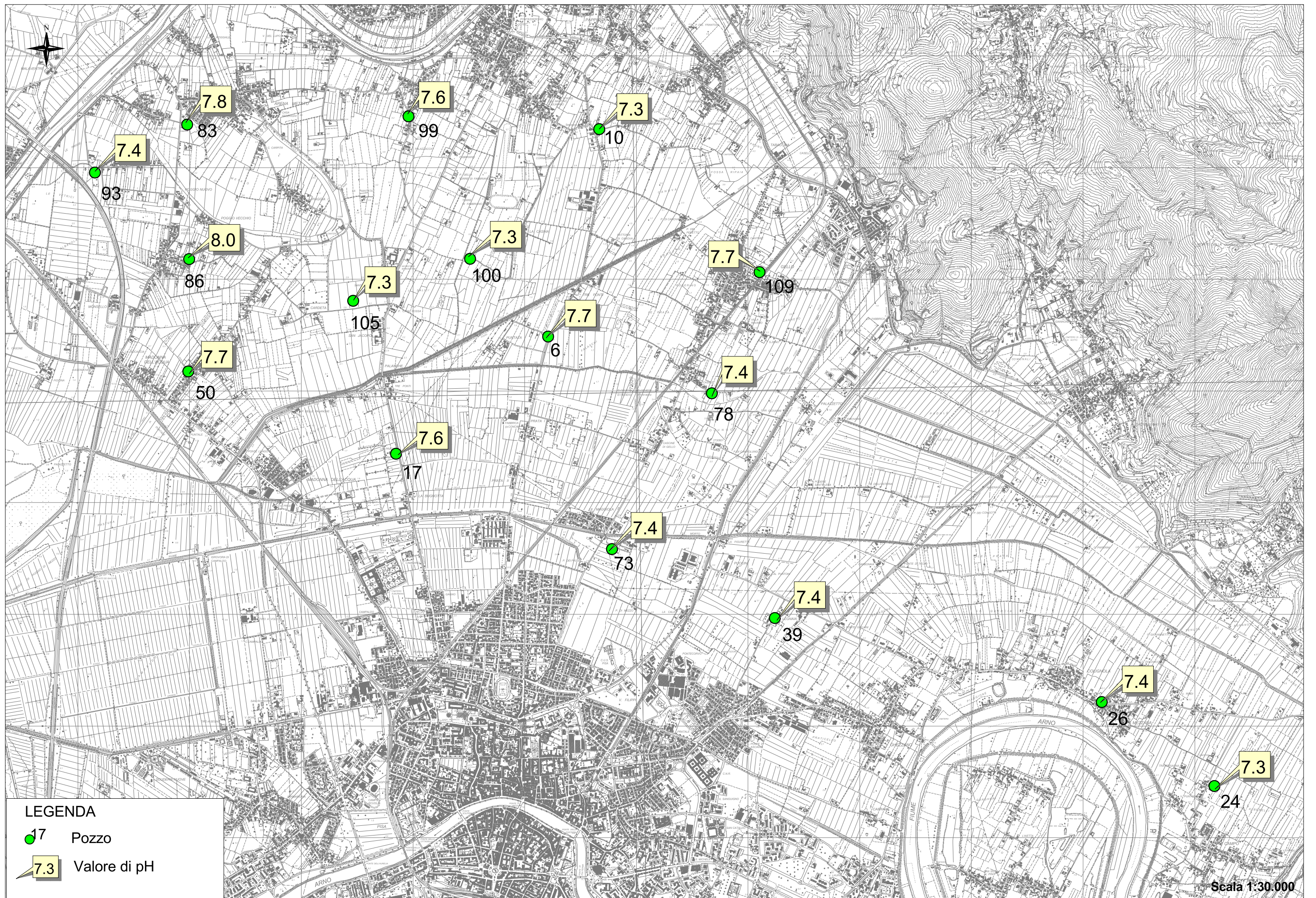
Tavola 3 - Ubicazione dei pozzi censiti e valore di pH misurato nel mese di marzo 2009
